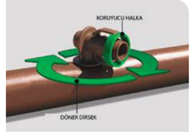
QF Damla Sulama Borusu Başlığı
